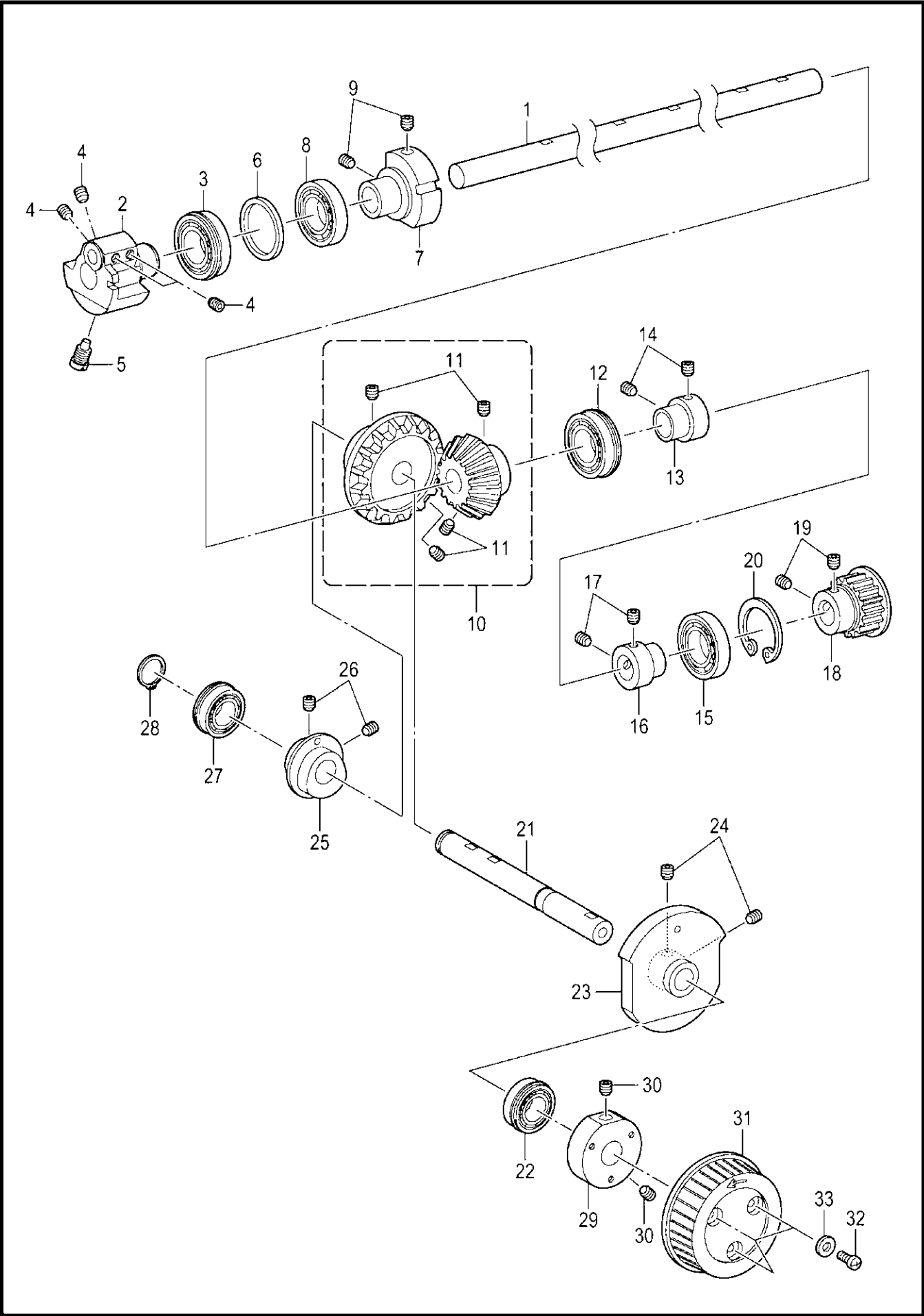
C . 上轴装置 / Upper shaft mechanism
