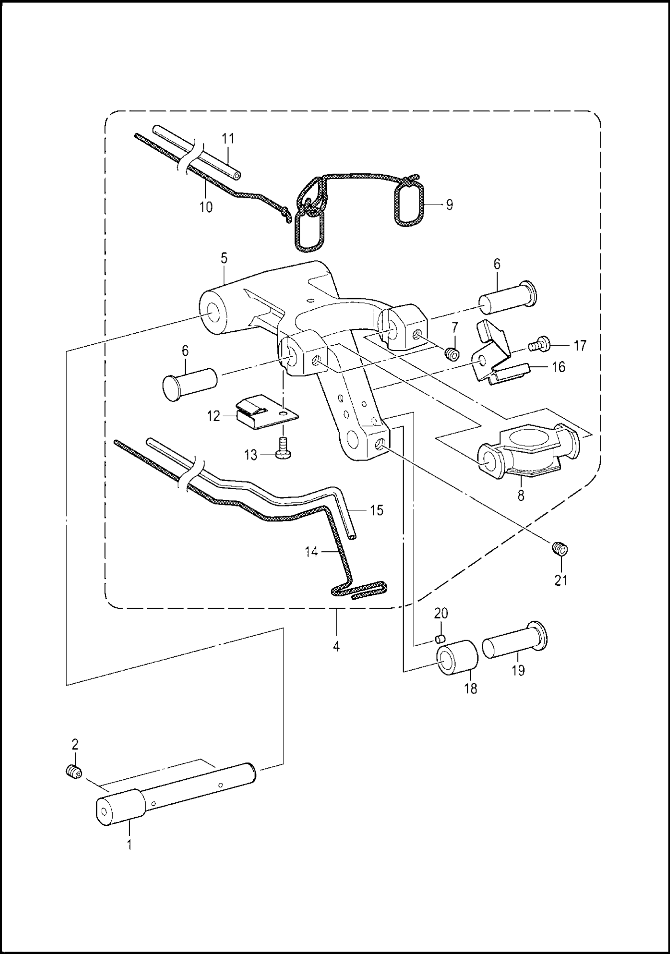
K. 弯针装置 / Looper mechanism
